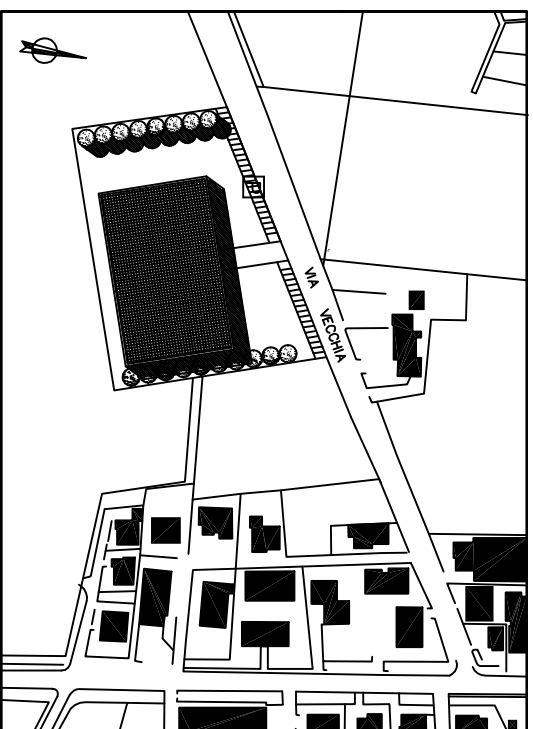
PLANIVOLUMETRICO Sc. 1:2000
